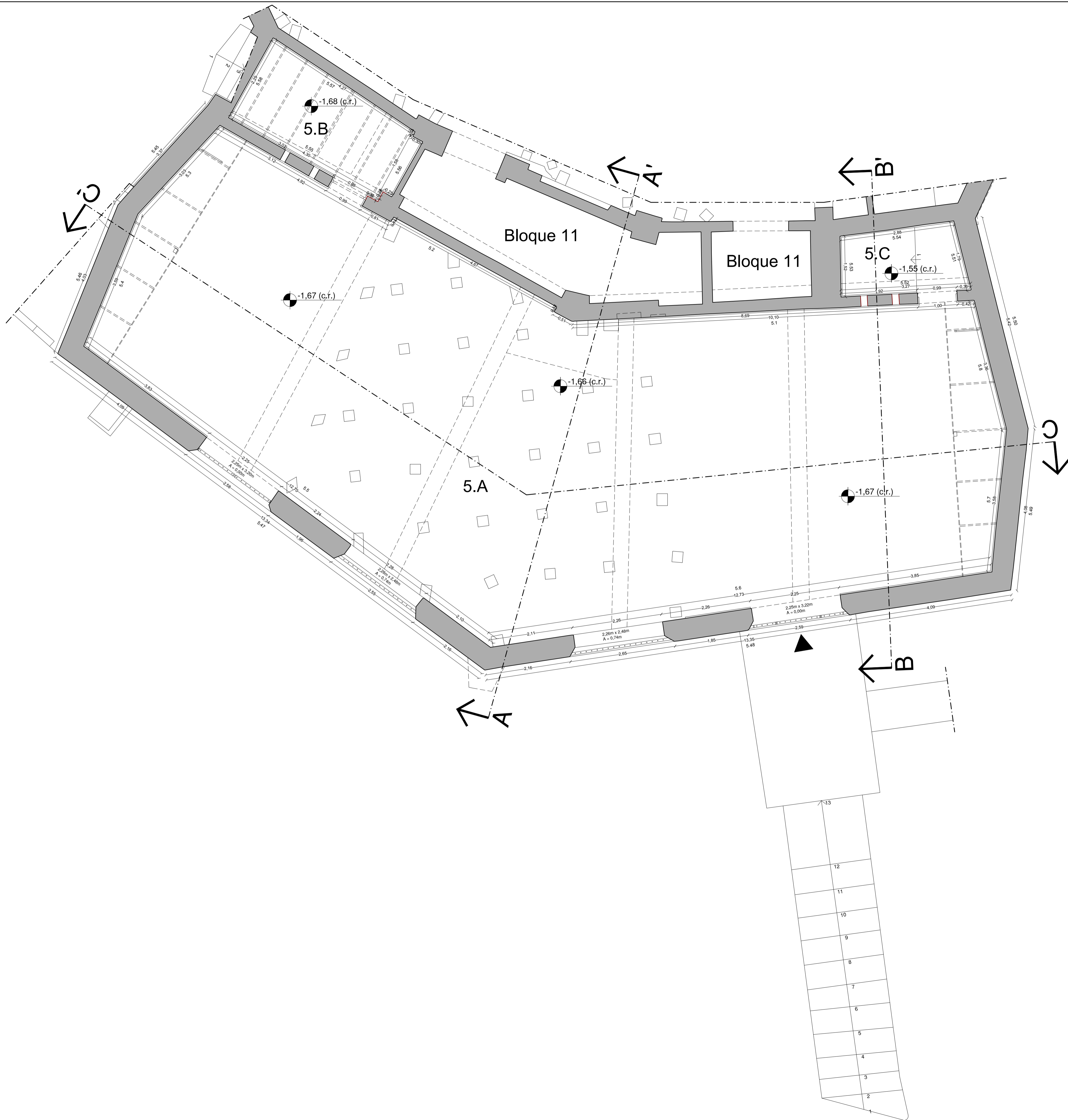
Planta a cota -0,38 (c.r.)
